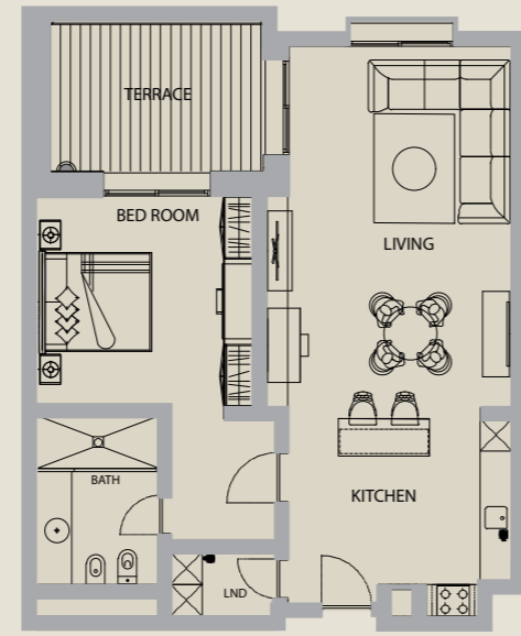
1 BED ROOM F1-12/F2-12 /F3-12 LEVEL: L1/L2/L3
